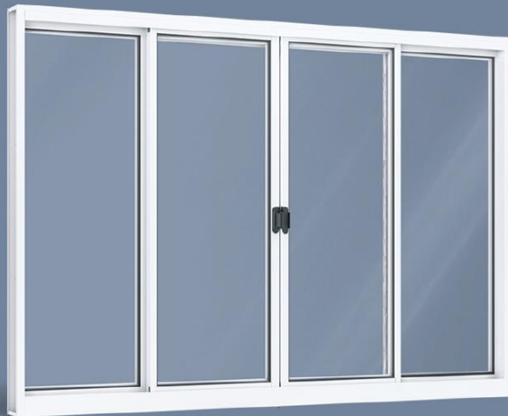
142. DE CORRER CENTRAL 2 FOLHAS MOVEIS E 2 FIXAS
