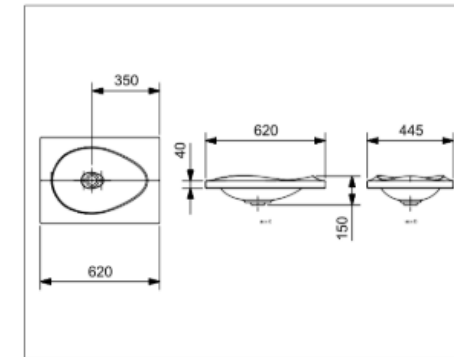
Desenho Técnico 620X445 Diseño Técnico 620X445
