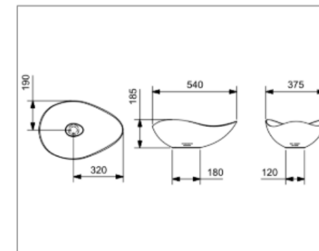
Desenho Técnico 540X375 mm Diseño Técnico 540X375 mm
