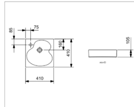
Desenho Técnico 410X410 mm Diseño Técnico 410X410 mm
